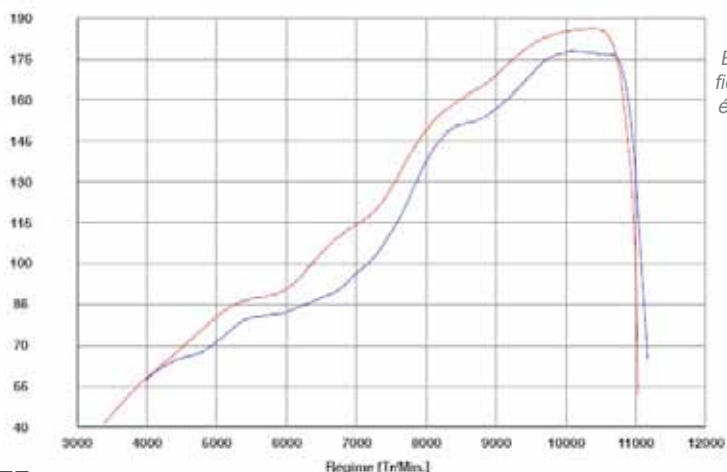
Puissance à la roue corrigé [CV]
